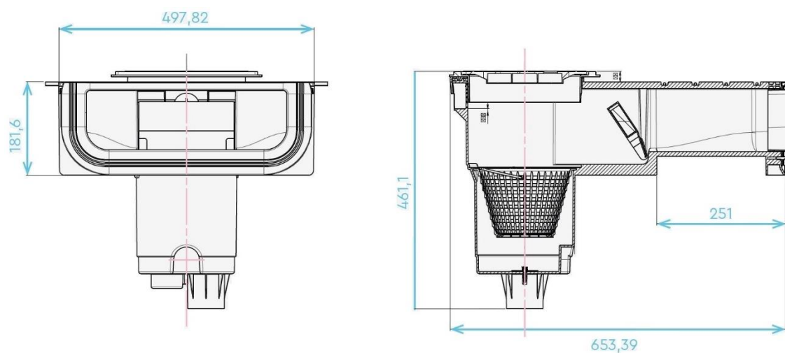
Cod. 1070271 - Skimmer sfioratore in ABS bianco con inserti in ottone per piscine in cemento
