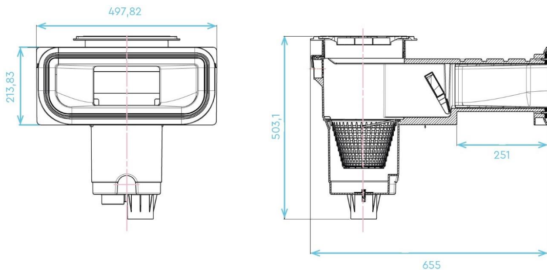
Cod. 1070270 - Skimmer in ABS bianco con inserti in ottone per piscine in cemento
