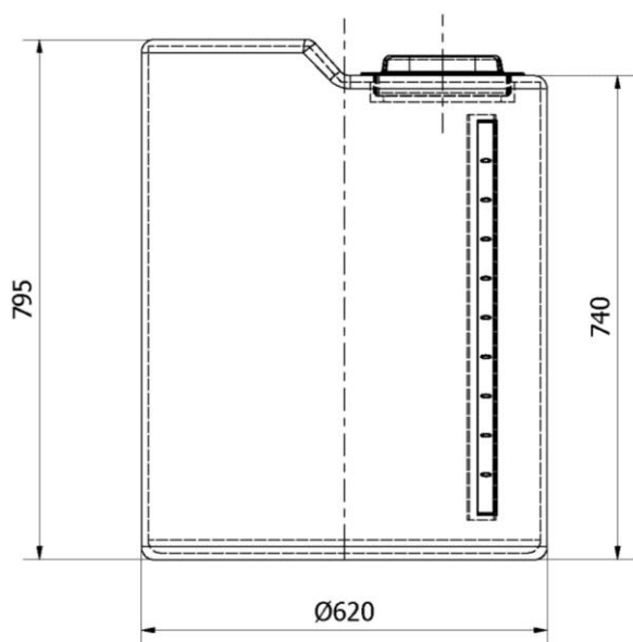
Contenitore di stoccaggio da 215 litri – Cod. 1075101
