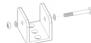
Cod. 1040348 Staffa a immersione Immersion bracket
