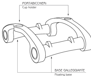
Cod. 1040349 Supporto galleggiante Floating base
