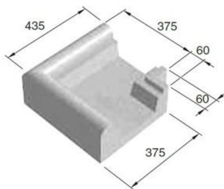
Angolo rovescio - Inverted Angle
