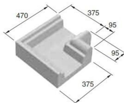
Angolo retto - Right Angle
