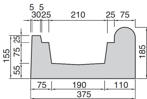
Sezione senza piletta - Section without waste
