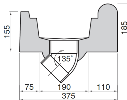
Sezione con piletta Ø100 - Section with Ø100 waste
